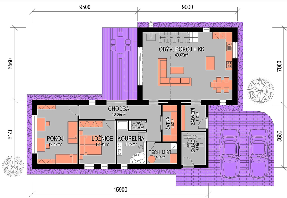
Přízemí - užitná plocha 125,70m 2
